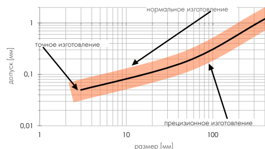
Рисунок 3: Допуски при обработке резанием материалов ZEDEX®.
