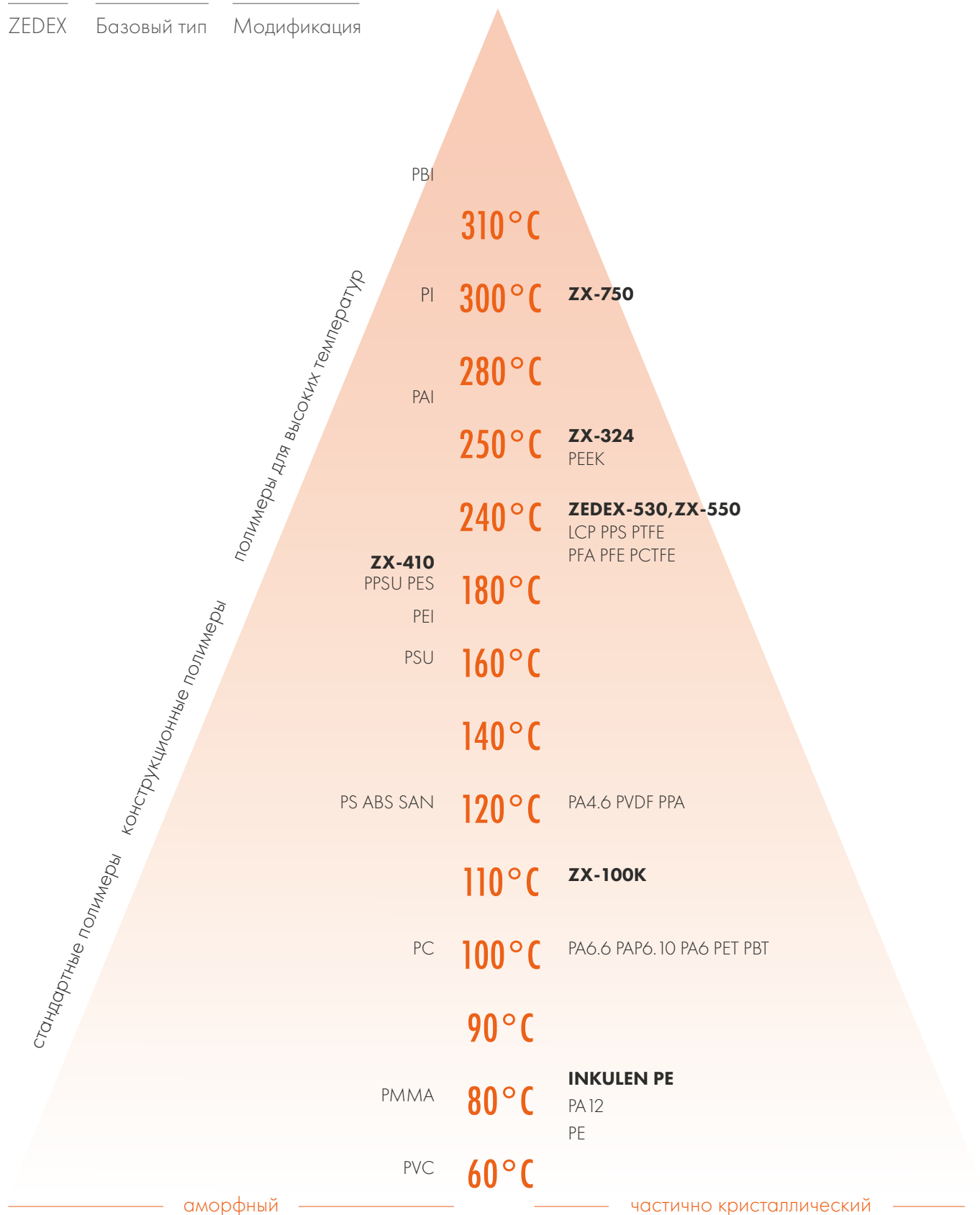
Рисунок 1: Температуры длительного применения базовых типов ZEDEX®.
