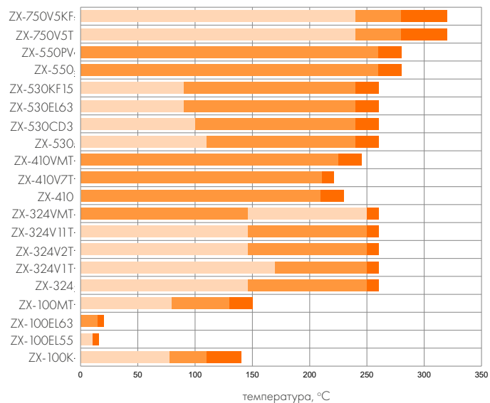
Рисунок 2: Температурные границы применения материалов ZEDEX®.
