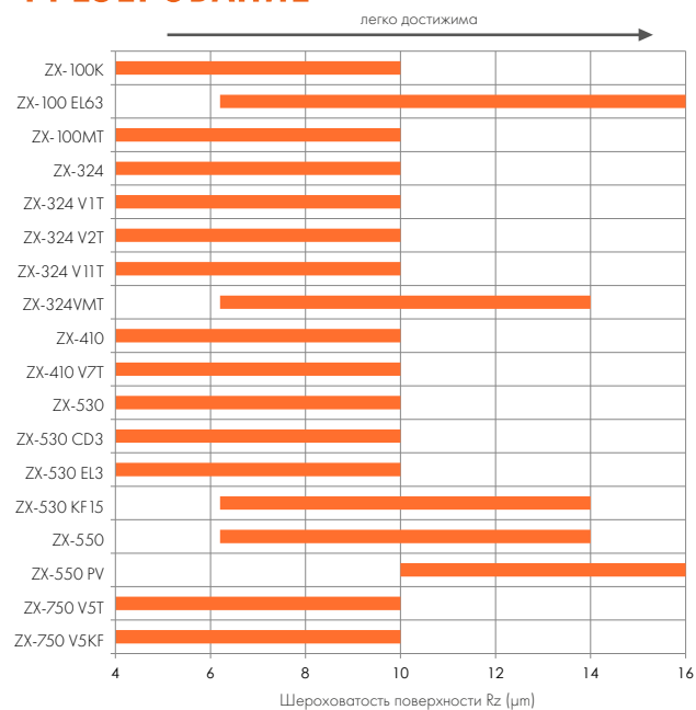
Рисунок 4: Достижимая шероховатость поверхности материалов ZEDEX®.
